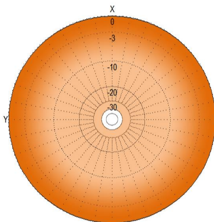
Lóbulo Horizontal
