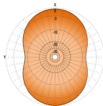
Lóbulo Horizontal
