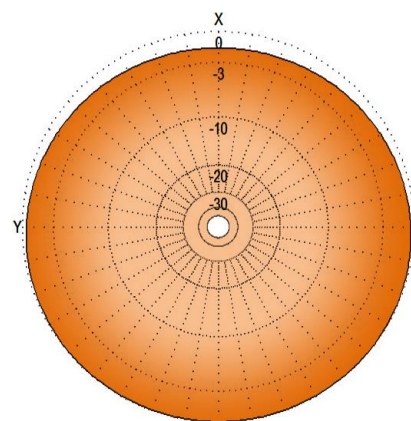
Lóbulo Vertical
