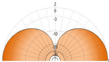
Lóbulos Vertical
