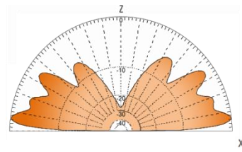
Lóbulo Vertical
