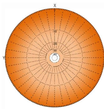
Lóbulo Horizontal
