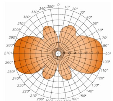
Lóbulo Vertical
