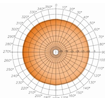
Lóbulo Horizontal
