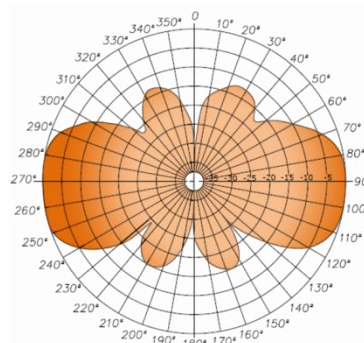
Lóbulo Vertical
