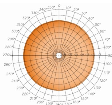
Lóbulo Horizontal
