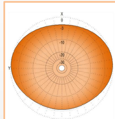
Lóbulo Horizontal*
