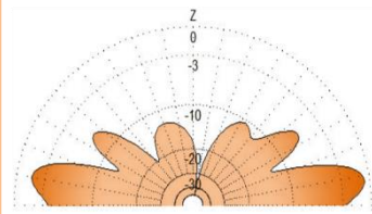
Lóbulo Vertical*
